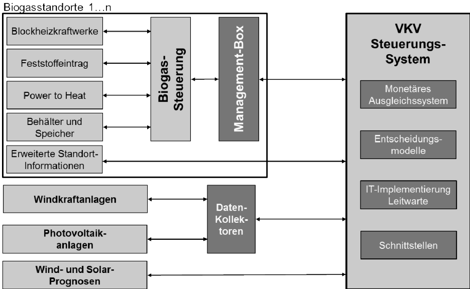
Abbildung 2: Aufbau des Steuerungssystems
